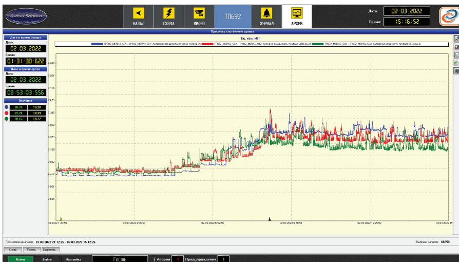
Рис. 2. График активной мощности по трем фазам
